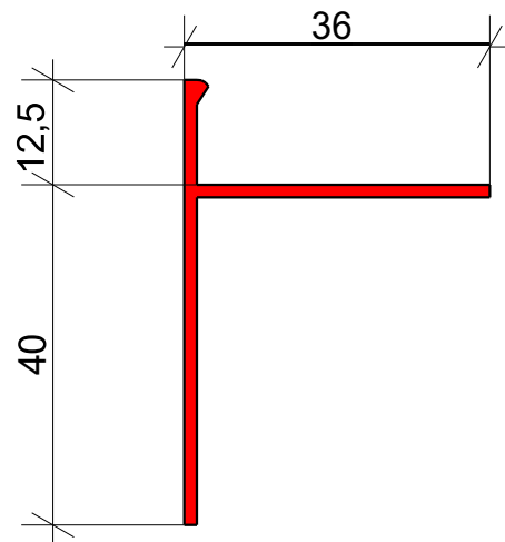
TERRASSENPROFIL 12,5 mm
