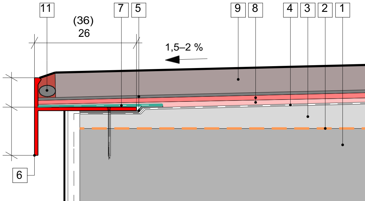
TERRASSENPROFIL 10 mm
