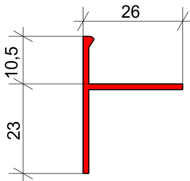
TERRASSENPROFIL 10 mm
