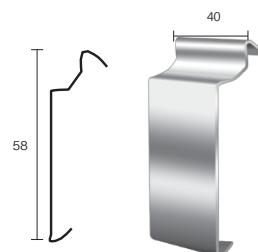
Verbindungsstück – GERAD/FLEXI Material: Al
