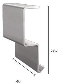
Verbindungsstück – RT/60 mm Material: Al
