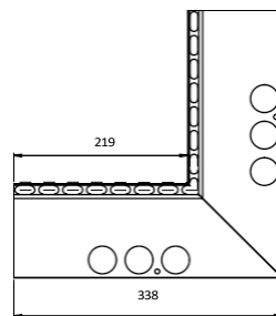
Eckstück – RT/60 mm Material: Al
