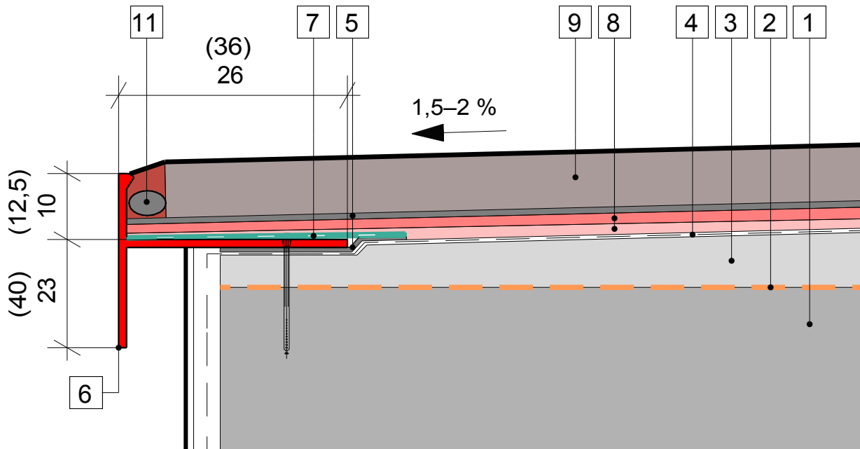
TERRASSENPROFIL 10 mm
