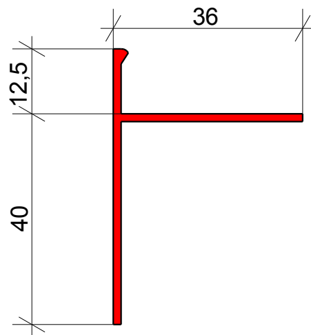
TERRASSENPROFIL 12,5 mm
